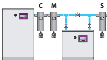
Třída 1-4-1 Filtrace před kondenzační sušičkou, kondenzační sušička a jemná filtrace od oleje a pevných nečistot.
