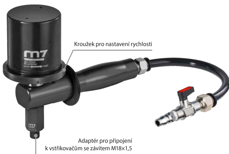
SC-0320 vyklepávač vstřikovačů paliva v sadě
