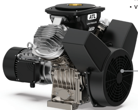
ATL-2,2-T 2,2 kW, samostatná jednotka
