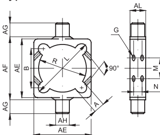
Centre trunnion (profile barrel) MT4 for cylinders AMB
