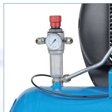
Dvojitý výstup pro možnost odběru vzduchu pro dvě pracovní aplikace najednou
